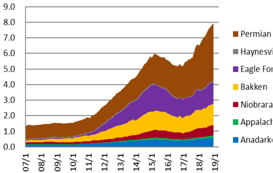
(単位: 百万) シェールオイル主要鉱区 生産量
